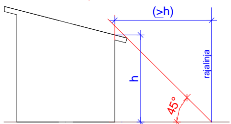
Päätyräystäs rajan suuntaan
